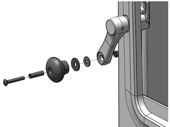
Afb. 3b Installatie van de deurhendel (F 205 - modern)
