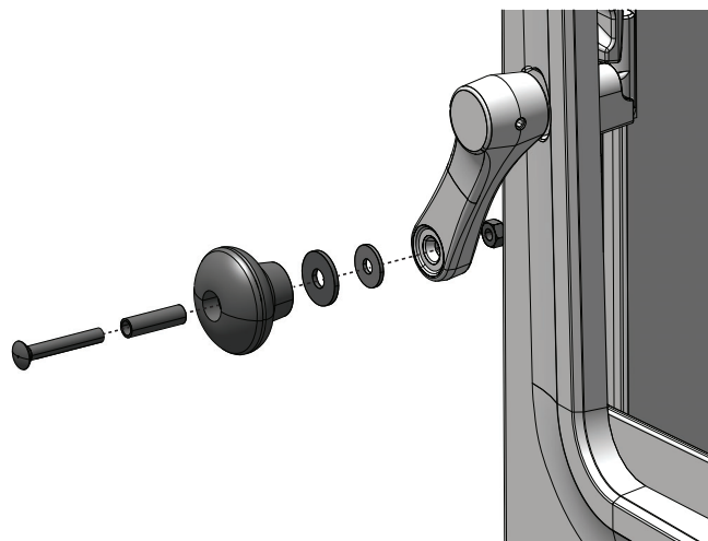
Rys. 3b Montaż klamki (F 200 - nowoczesna)
