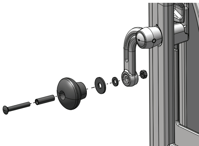
Rys. 3a Montaż klamki (F 200 - klasyczna)
