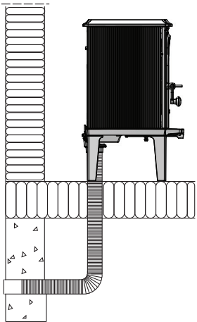
Afb. 6d Indirect via een buitenmuur
