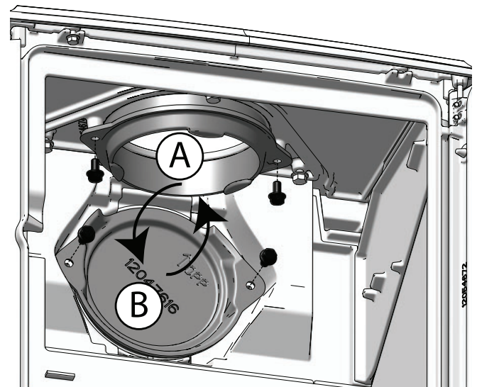
Afb. 4a Wisselen van bovenuitlaat naar achteruitlaat
