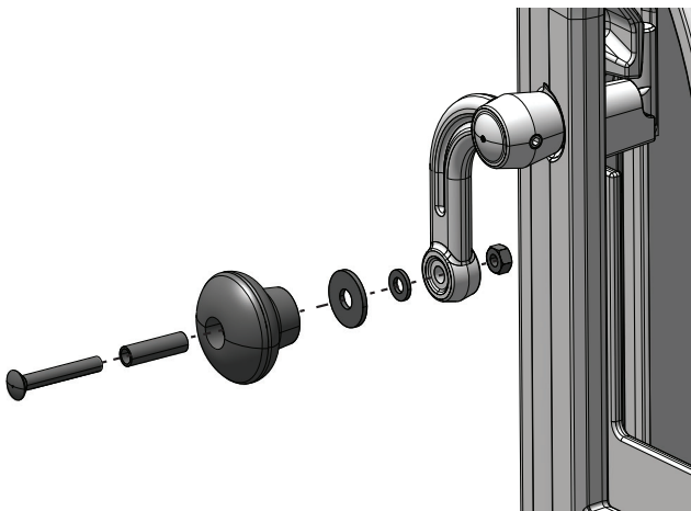
Afb. 3a Installatie van de deurhendel (F 200 - klassiek)
