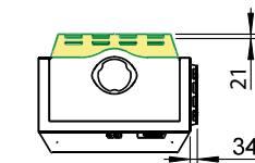
Konvektionsset, hinten
