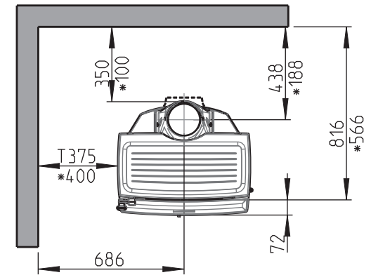
Mindestabstand zu brennbarer Wand
