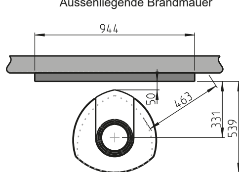
Aussenliegende Brandmauer
