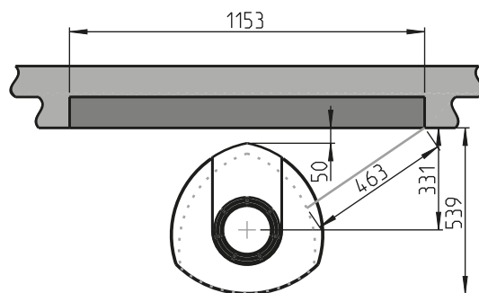
Eingebaute Brandmauer
